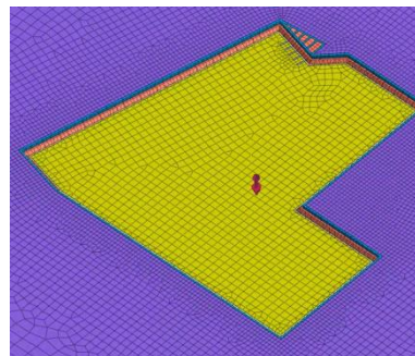
第二階段開挖(-9.7m)&扶壁移除
