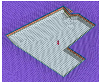
第二階段開挖(-9.7m)&扶壁移除
