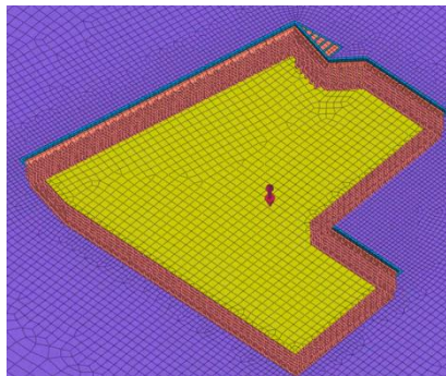
地改壁施作-內側
